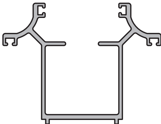
COLUMNA PRINCIPAL Perfil: 4363 Peso: 0,988 Kg/m
