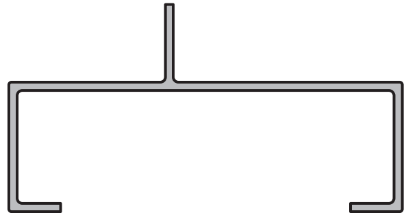
CANAL CON UNA ALETA 76 x 25 x 1,6 mm.
