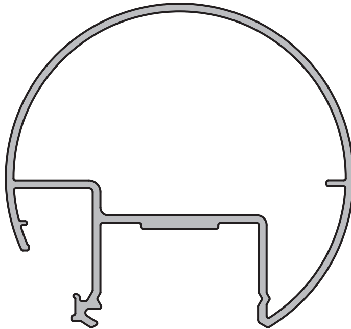
PASAMANOS 90 mm Perfil 7988 Peso: 1,941 kg/m
