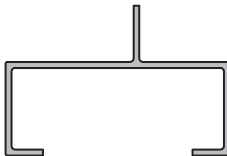
CANAL CON UNA ALETA DE 60 x 25 x 1,6 mm.
