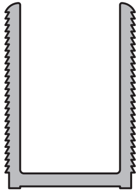
U DE ARMADO SERIE 90 x 40 x 2 mm. Perfil: 3022 Peso: 1,188 Kg/m
