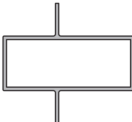
TUBO RECTANGULAR CON DOS ALETAS DE 60 x 25 x 1,6 mm.
