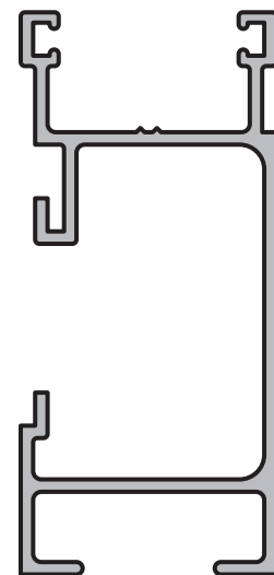
ZOCALO PASACABLE Perfil: 4365 Peso: 0,832 Kg/m
