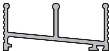
UMBRAL Perfil: 31 Peso: 0,510 Kg/m Matriz: M0724
