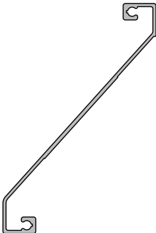
PARASOL DE ALETA FIJA Perfil: 5650 Peso: 0,780 Kg/m
