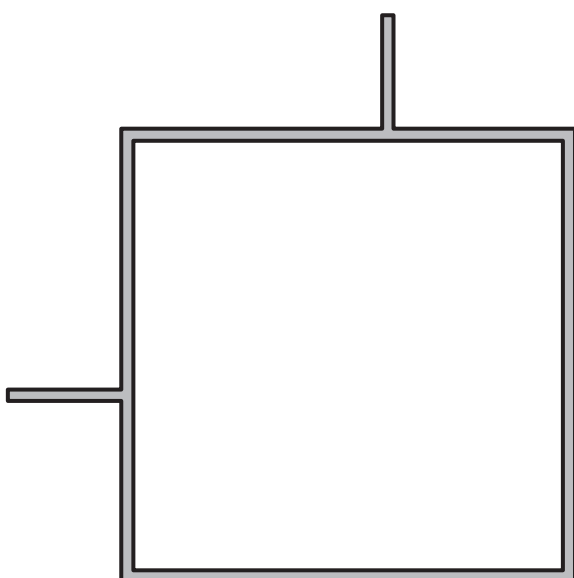
TUBO CUADRADO CON DOS ALETAS DE 60 x 1,6 mm.
