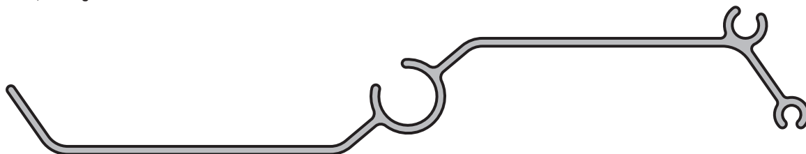
PARASOL DE ALETA FIJA Perfil: 5650 Peso: 0,780 Kg/m
