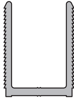
U DE ARMADO SERIE 90 x 40 x 1,5 mm. Perfil: 494 Peso: 1,237 Kg/m Matriz: M1982
