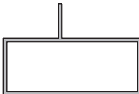
TUBO RECTANGULAR CON UNA ALETA DE 60 x 25 x 1,6 mm.
