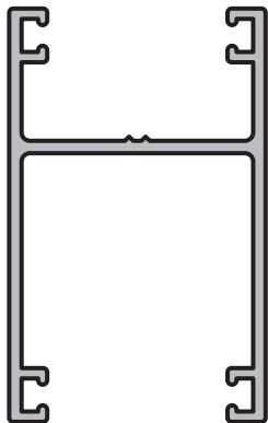
TRAVESAÑO Perfil: 4361 Peso: 0,620 Kg/m
